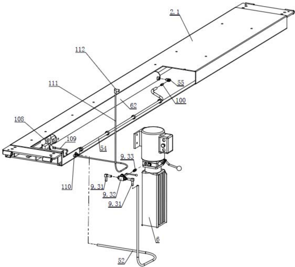
EHF9A 液压连接爆炸图
